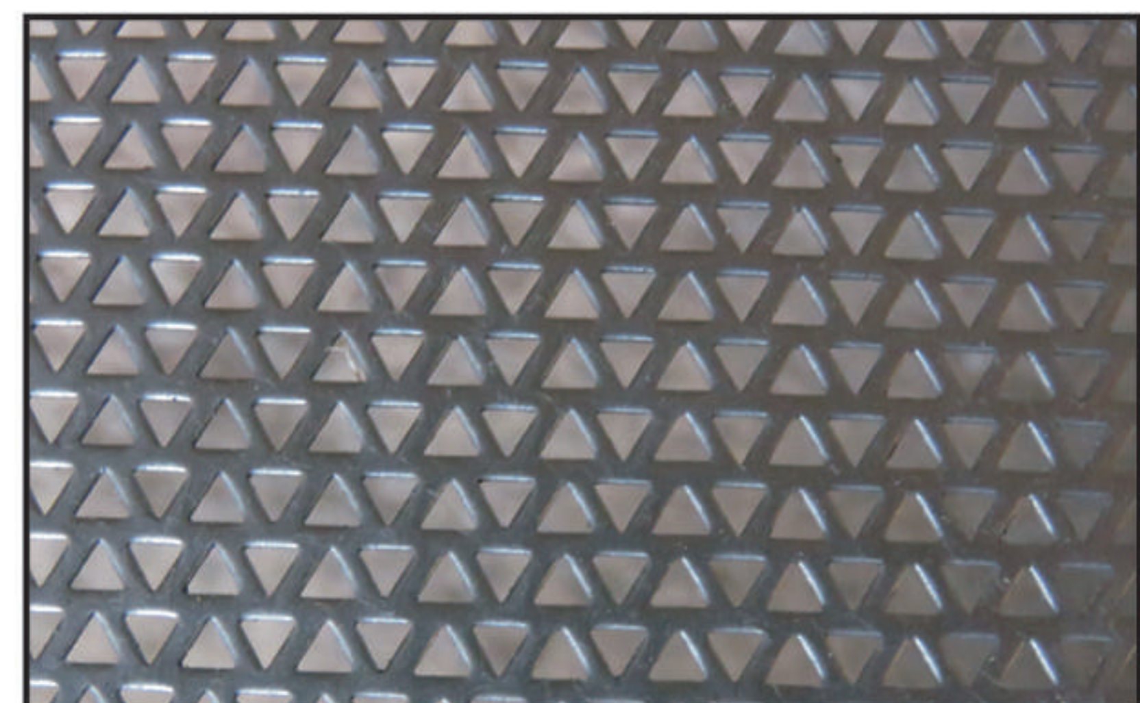
توری مثلثی بوجاری Triangular Hole 3-3/5 (mm)
