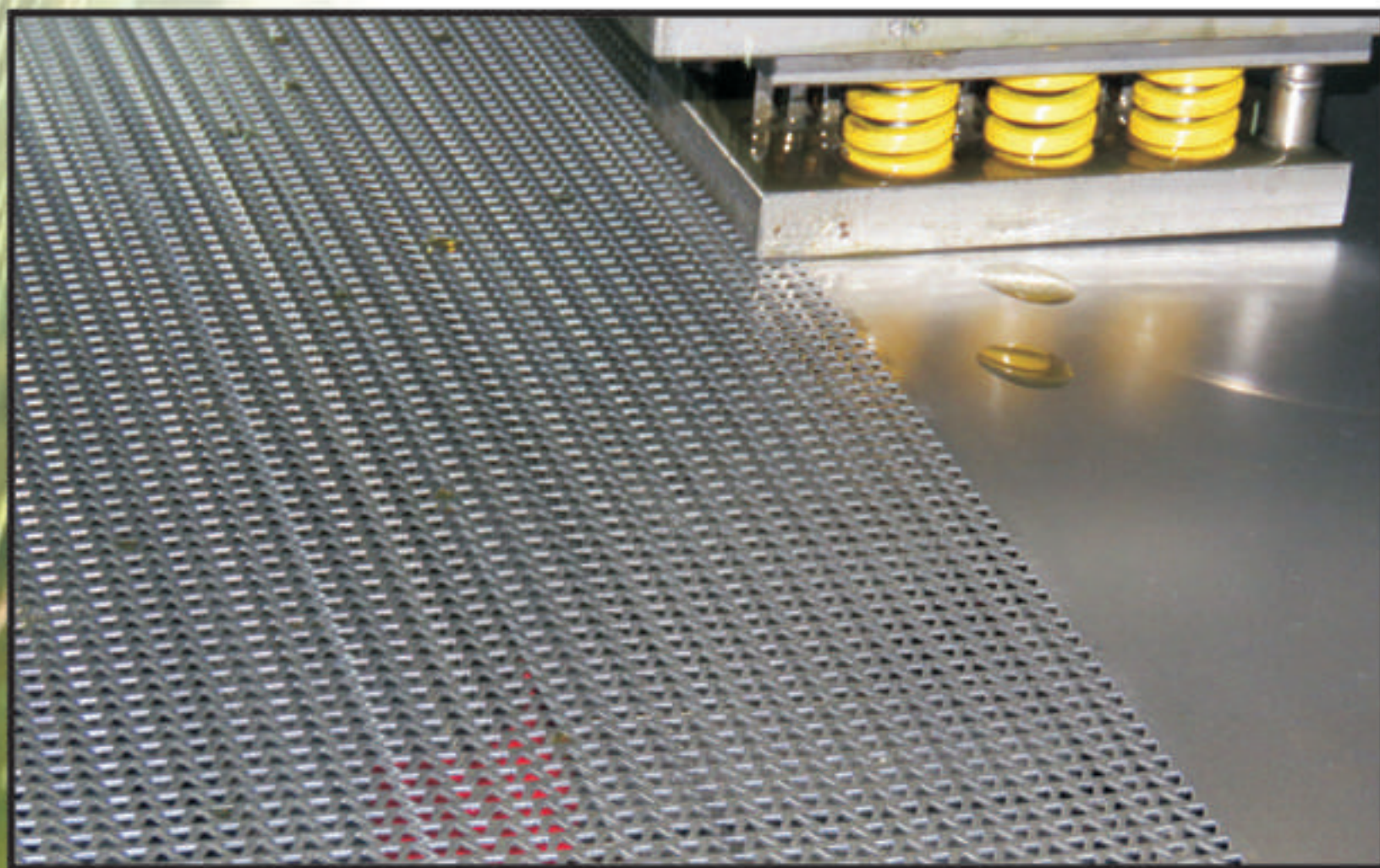
انواع توری های گرد بوجاری Round Hole
